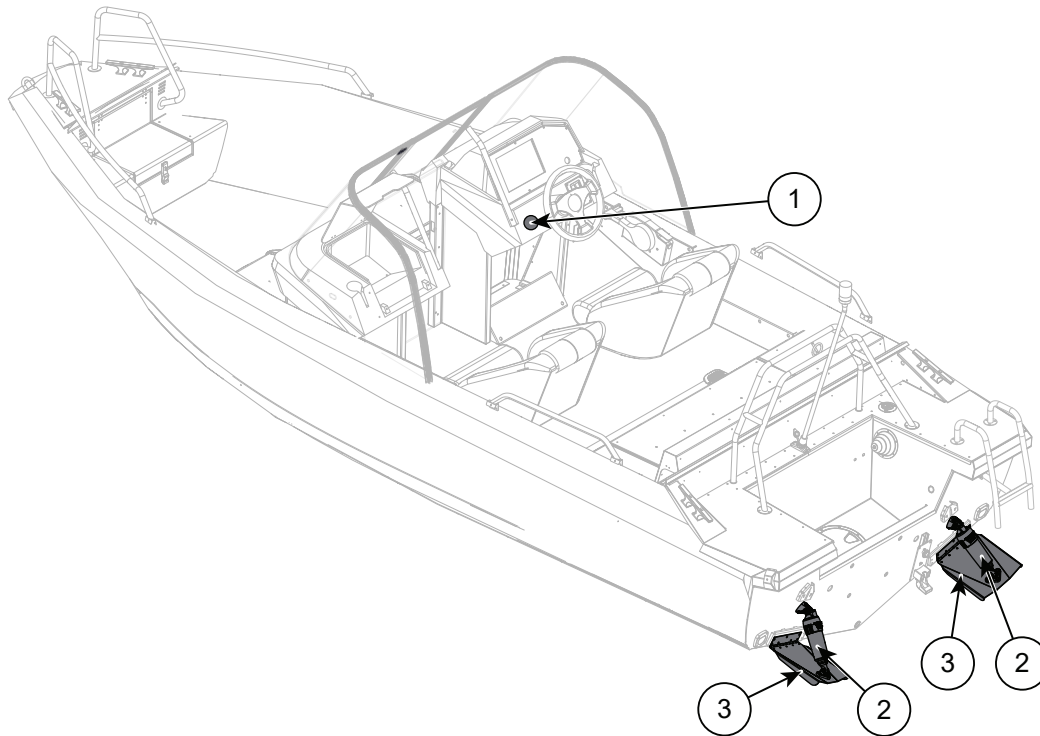
Kuva 5.4 Buster X:n trimmijärjestelmän komponentit
