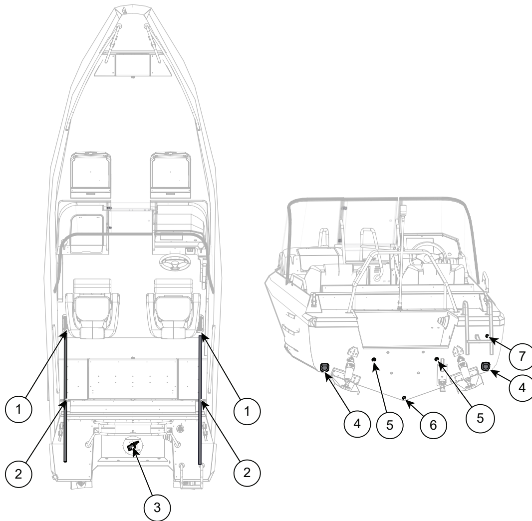
Kuva 9.1 Buster X:n tyhjennysvarustus
