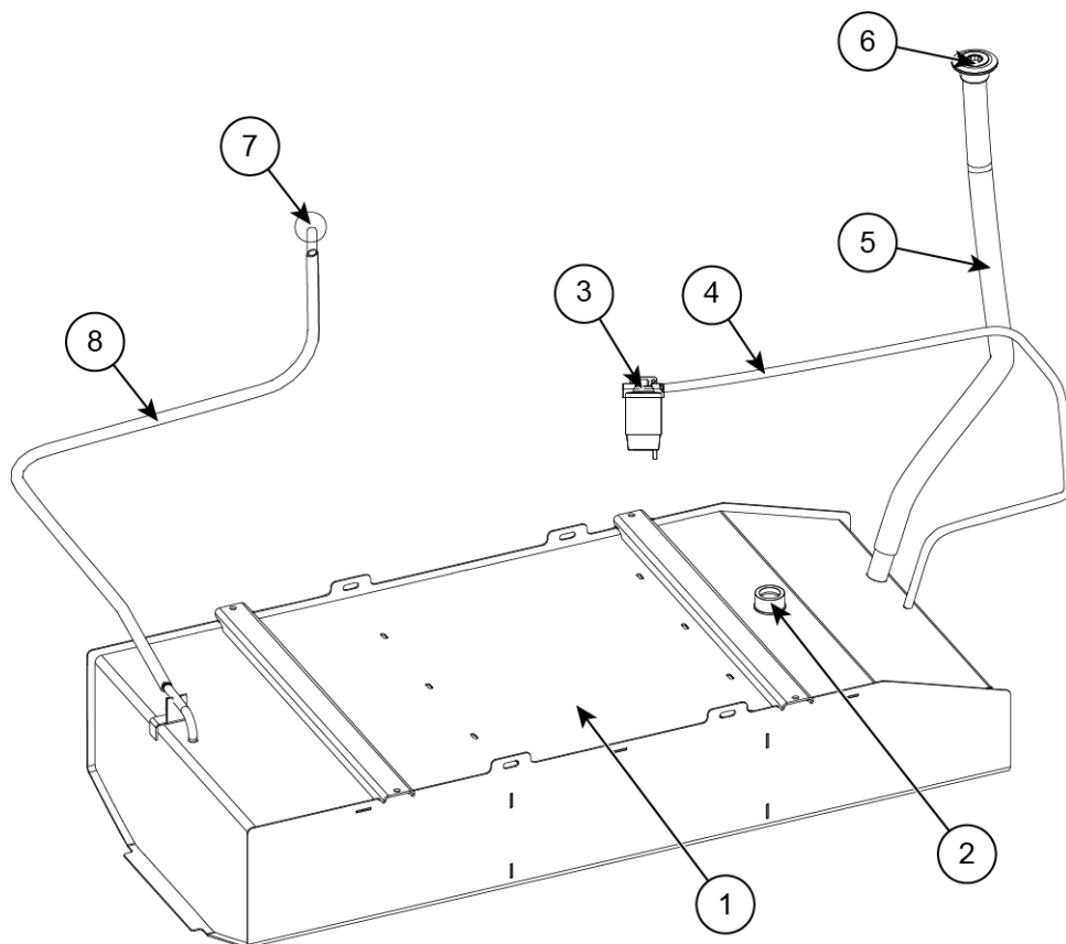
Kuva 6.1 Polttoainejärjestelmä
