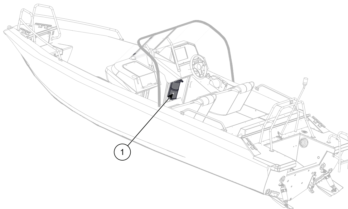
Kuva 2.2 Buster X:n palosammuttimen sijainti
