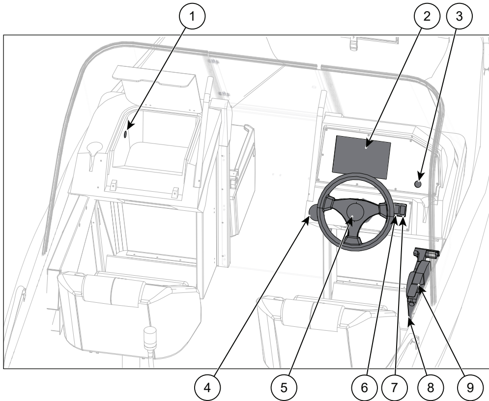
Kuva 5.1 Buster X:n ohjauspisteen hallintalaitteet
