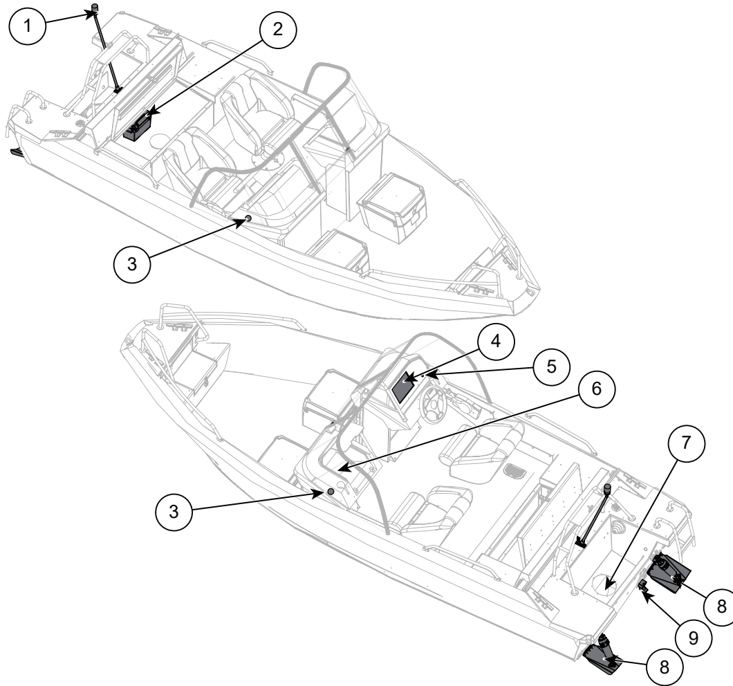
Kuva 8.2 Buster X:n sähkölaitteet
