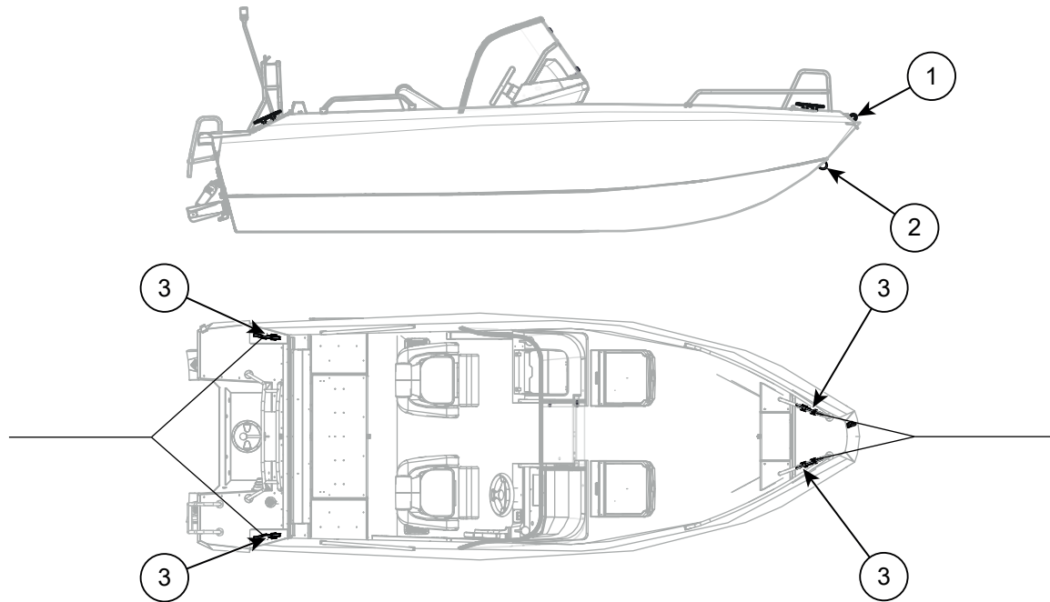
Kuva 5.5 Buster X:n kiinnitys- ja hinauspisteet
