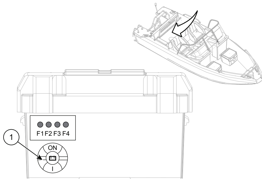
Kuva 8.1 Buster X:n päävirtakytkin ja sulakepaneeli
